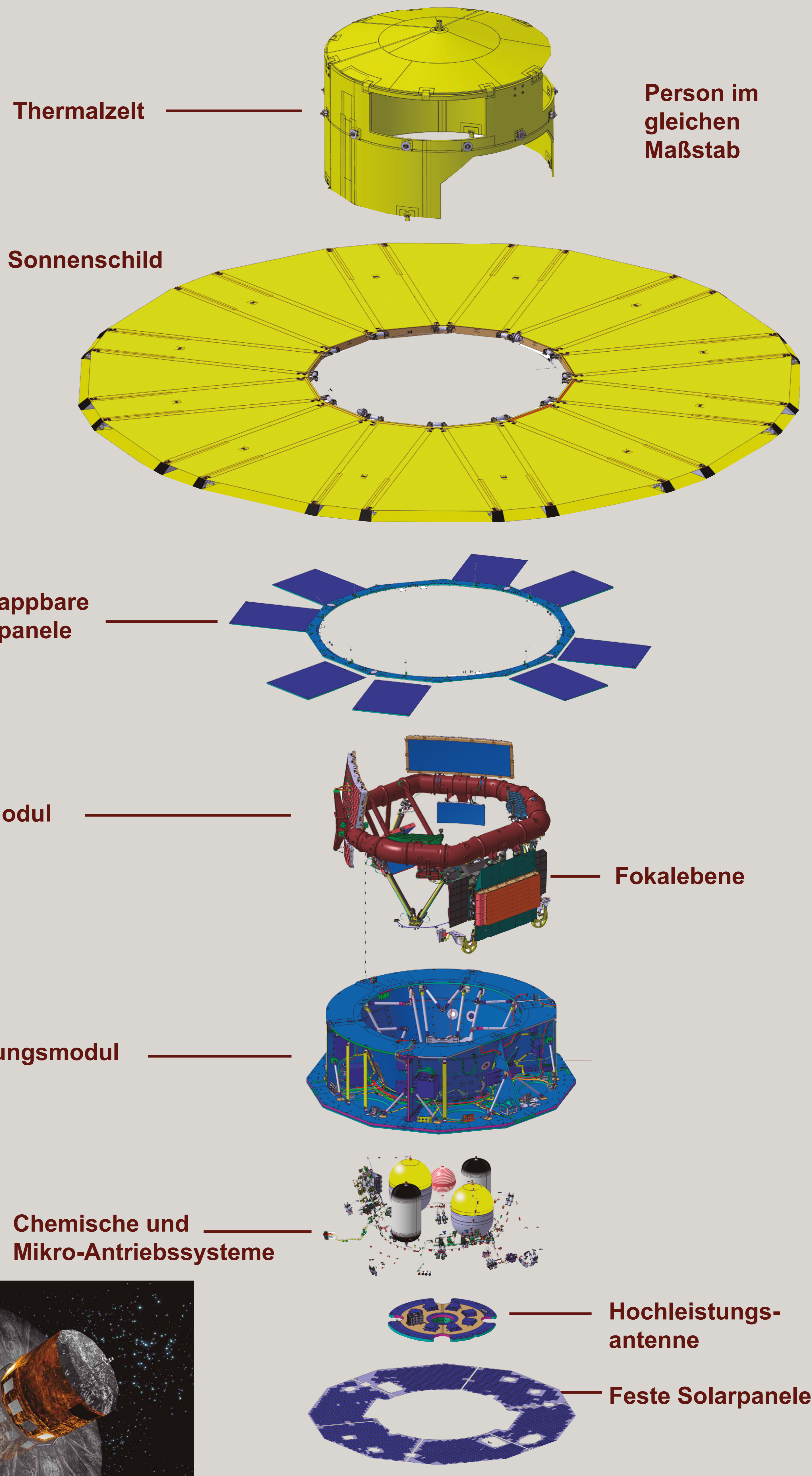
Aufbau des Gaia-Satelliten (ASTRIUM)
